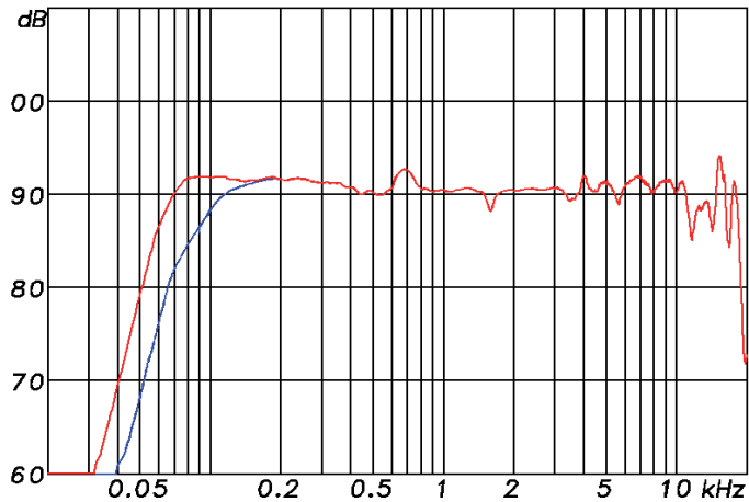
F 8 A hor. Direktivität Plot
