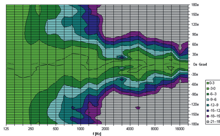
F 8 A vert. Direktivität Plot
